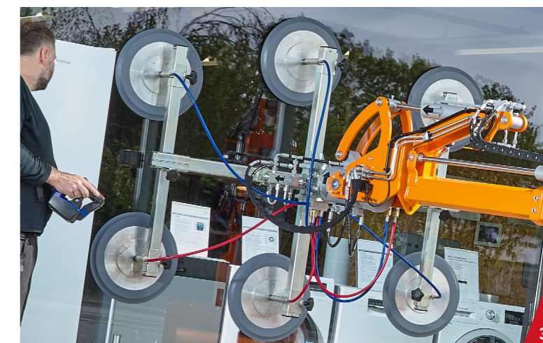
1 De SL809 is voorzien van 6 zuignappen met een doorsnede van 400mm 2 De SL809 Outdoor heeft proportionele rijbediening. 3 De SL809 is standaard uitgerust met een roteerbare kop.
